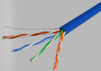
NCB-5EUGRYR-305MET CAT5E UTP 24AWG SOLID CABLE 305m
